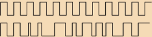
Fig. 1. Een word clock sigitaal met en zonder jitter
